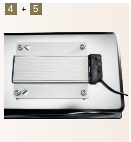
5 Elektro-Heizung Für Chafing Dishes mit Wasserbad Art.-Nr. 0740. Mit Regler. Anschlusswert: 230 V/700 Watt. Art.-Nr. 0889 €/Stück 79,99
